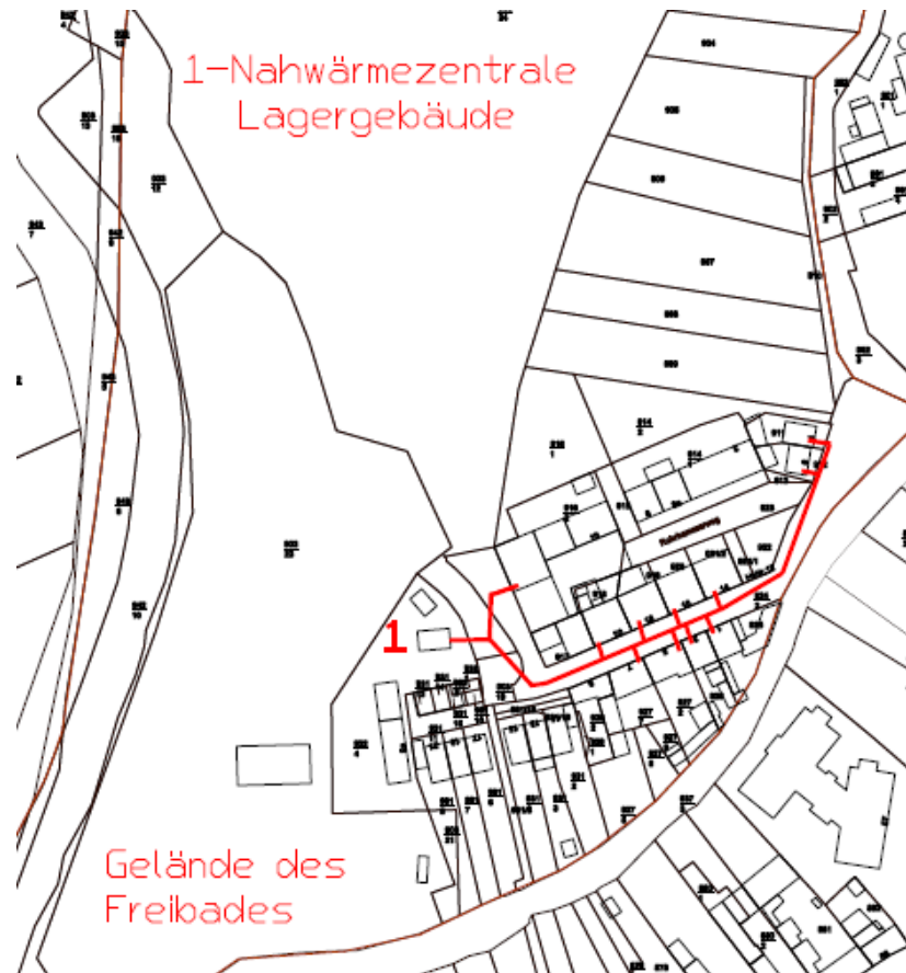
Bild: Schematischer Entwurf für ein mögliches Nahwärmenetz im Wohngebiet Rohrhammerweg
